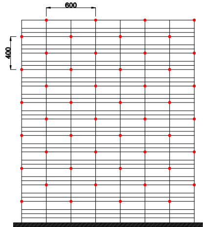
Disposition d'ancrages en configuration recouverte
