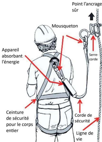
Utilisation du système d'arrêt de chute
