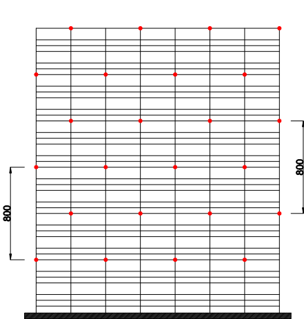
Disposition d'ancrages en configurations non-recouvertes
